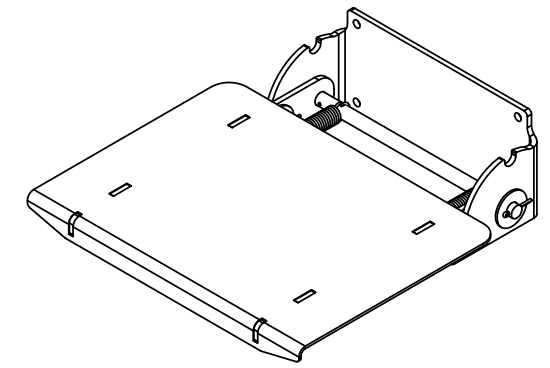
3-D VIEW SCALE: 1:8
